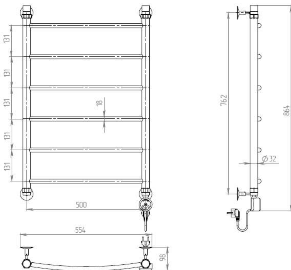
Водяной полотенцесушитель ДВИН Модель R Электро 800x500
